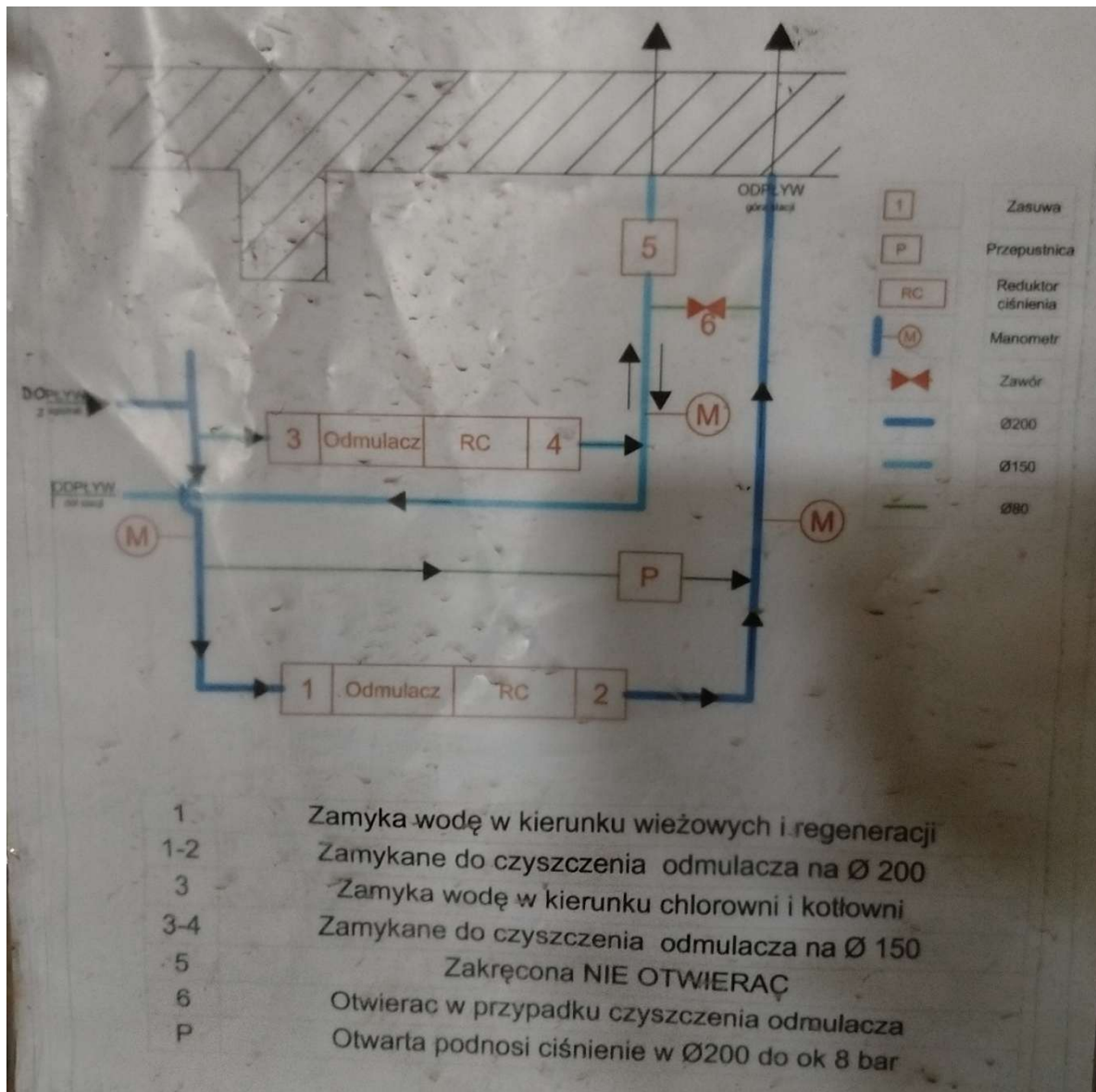
Schemat węzła reduktorów ciśnienia
